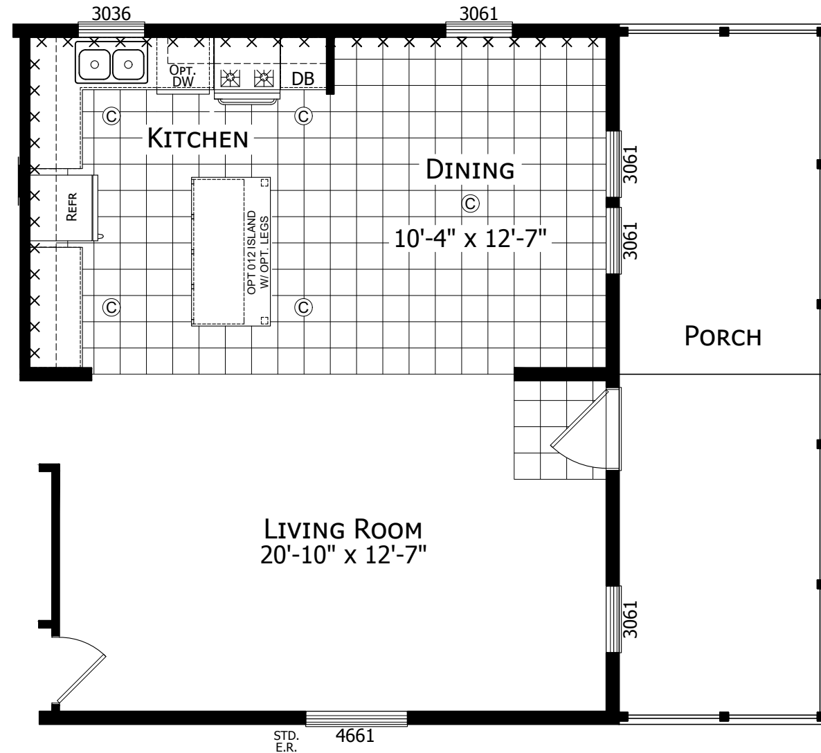
OPTIONAL PORCH
