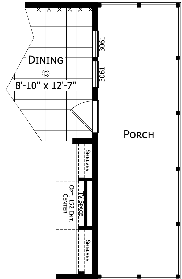
OPTIONAL PORCH
